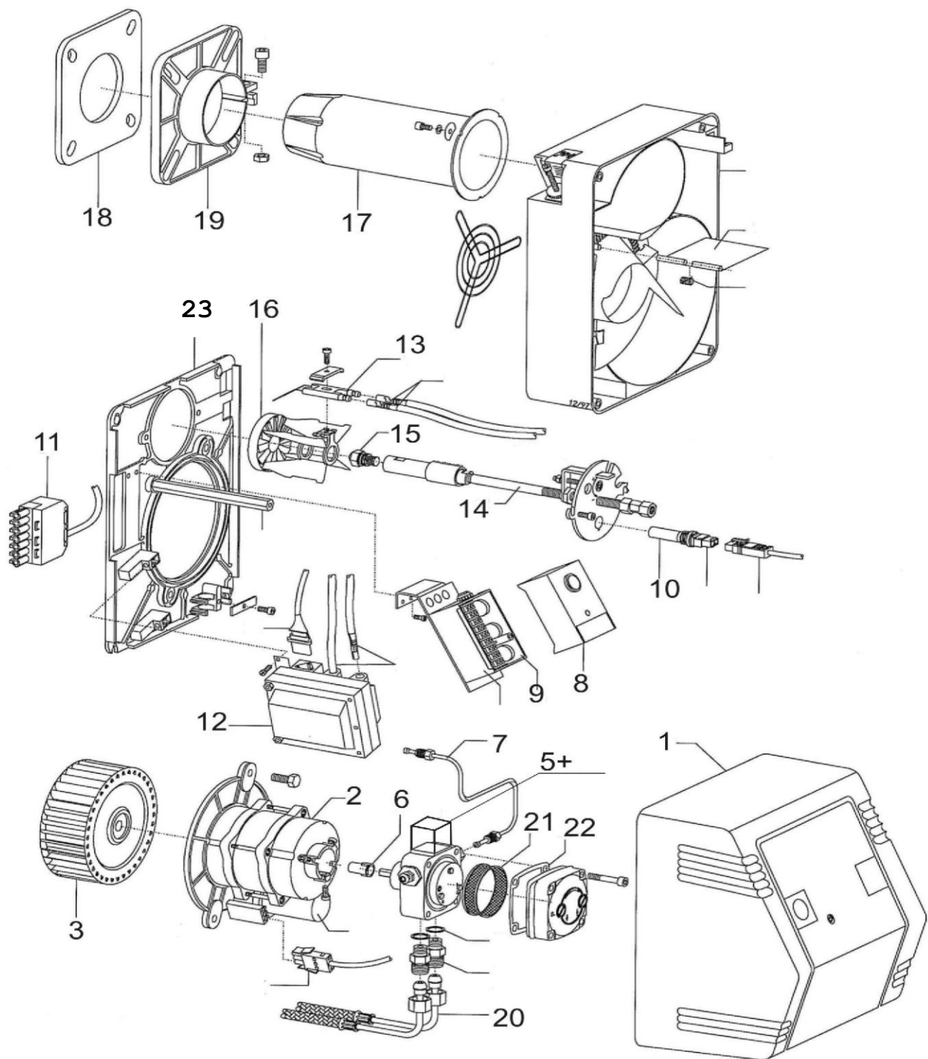
SLV 22/44/55 Brander/Burner/Bruleur/Brenner
